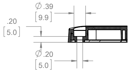
SECTION A-A SCALE 1 : 2
